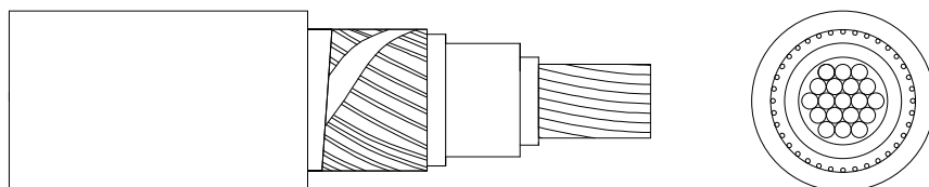
X-VOLT® HEPRZ1 18/30 kV
