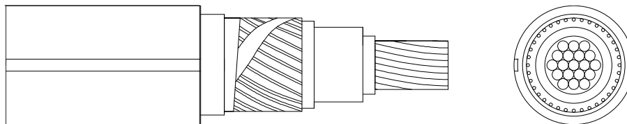
X-VOLT® RHZ1 (AS) 12/20 kV
